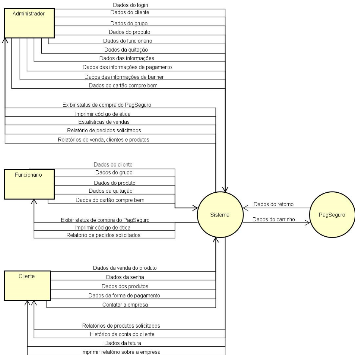
Diagrama 1 – Exemplo de diagrama de contexto
