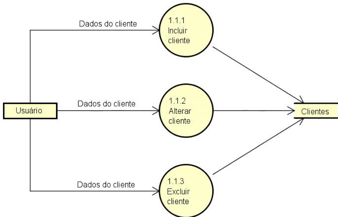
Diagrama 4 - DFD Nível 3 – Cadastrar Cliente
