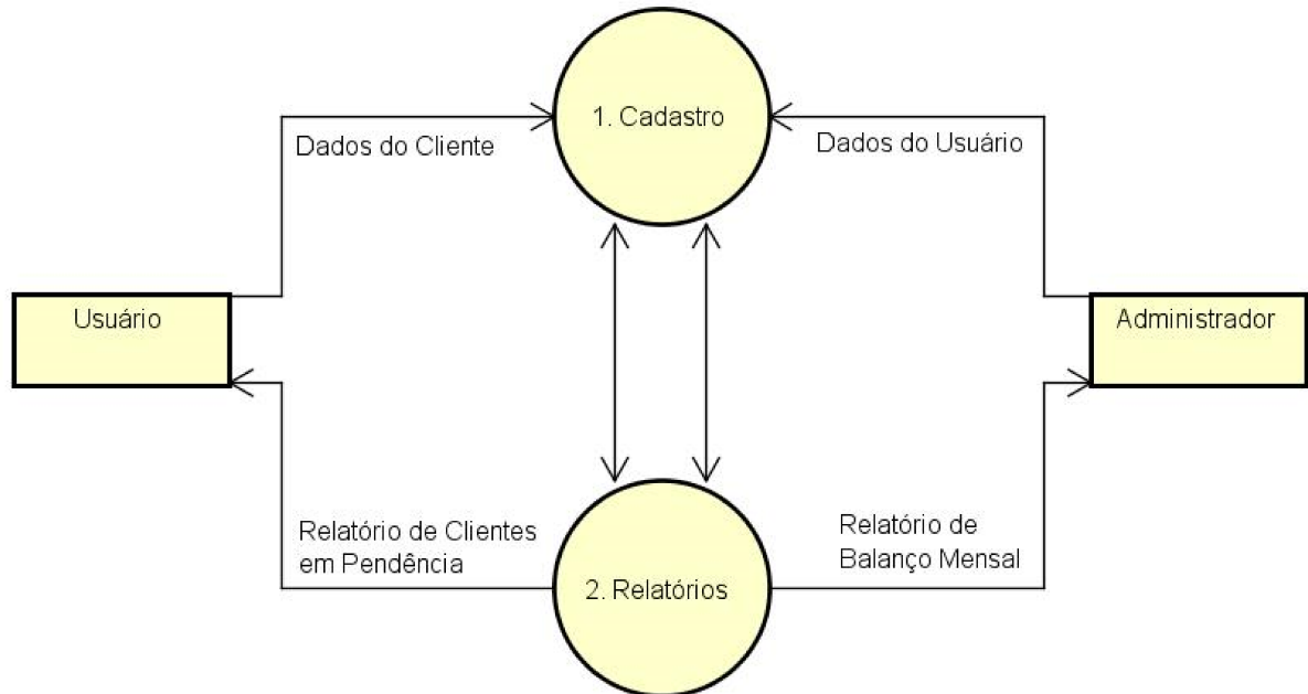
Diagrama 2 – Exemplos de diagrama de fluxo de dados – DFD nível 1
