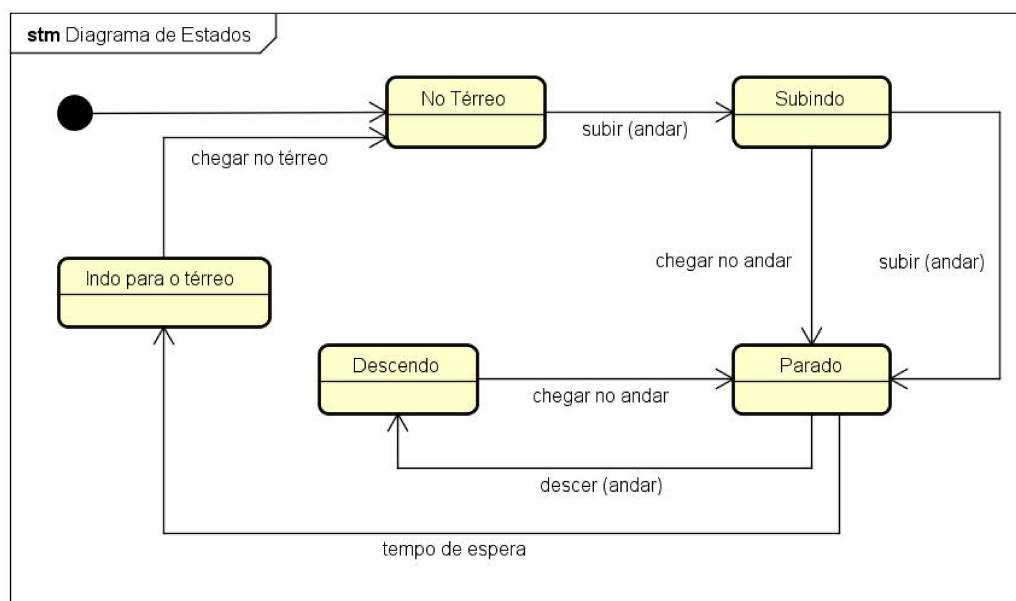
Diagrama 13 – Exemplo de diagrama de estados (statechart)
