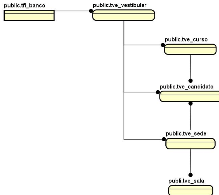
Diagrama 5 - Exemplo de diagrama de entidades e relacionamentos
