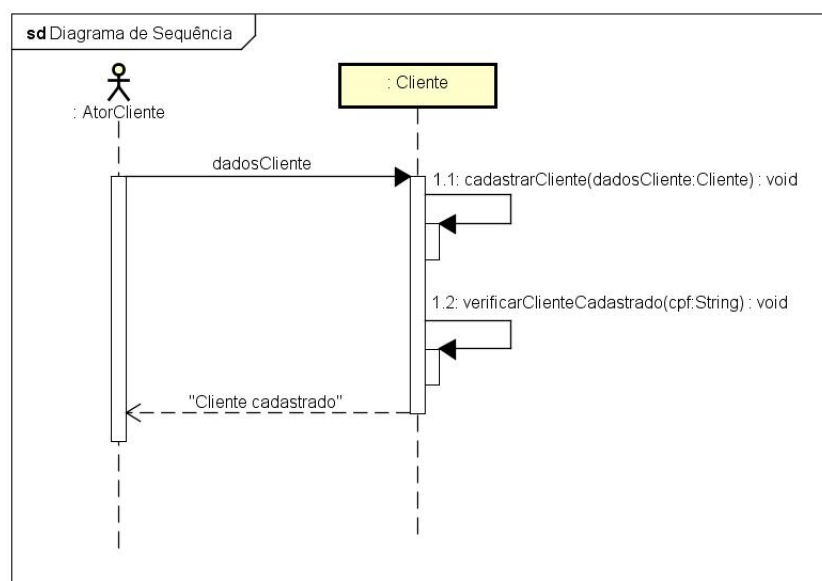
Diagrama 10 – Exemplo de diagrama de sequência
