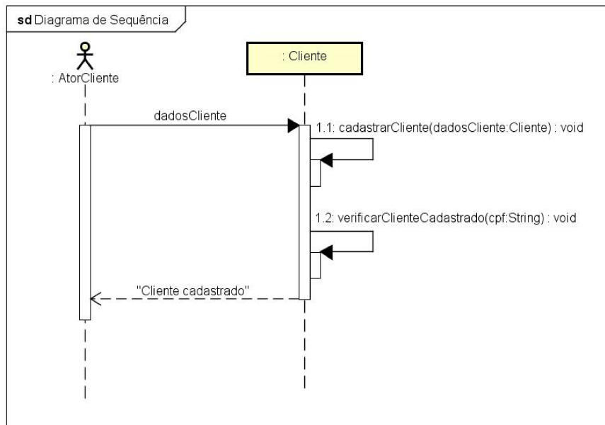
Diagrama 12 – Exemplo de diagrama de sequência
